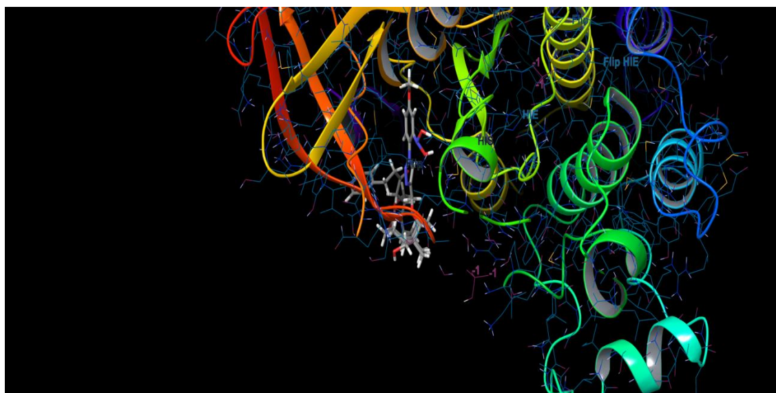
Ligand: 11
